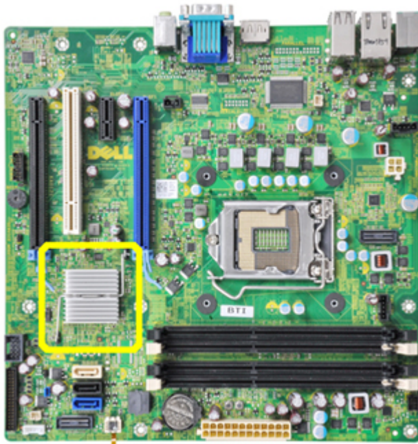
Figur 1. Bundkort af en tidligere version af bundkortet med kølelegeme
